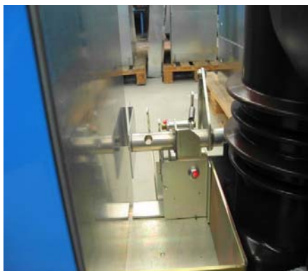
Foto 10: Boring in hoofdas ar-killer
